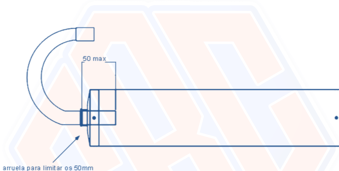
Figura 12 - Desenho Técnico referente ao ARTIGO 37º, PARÁGRAFO 12º
