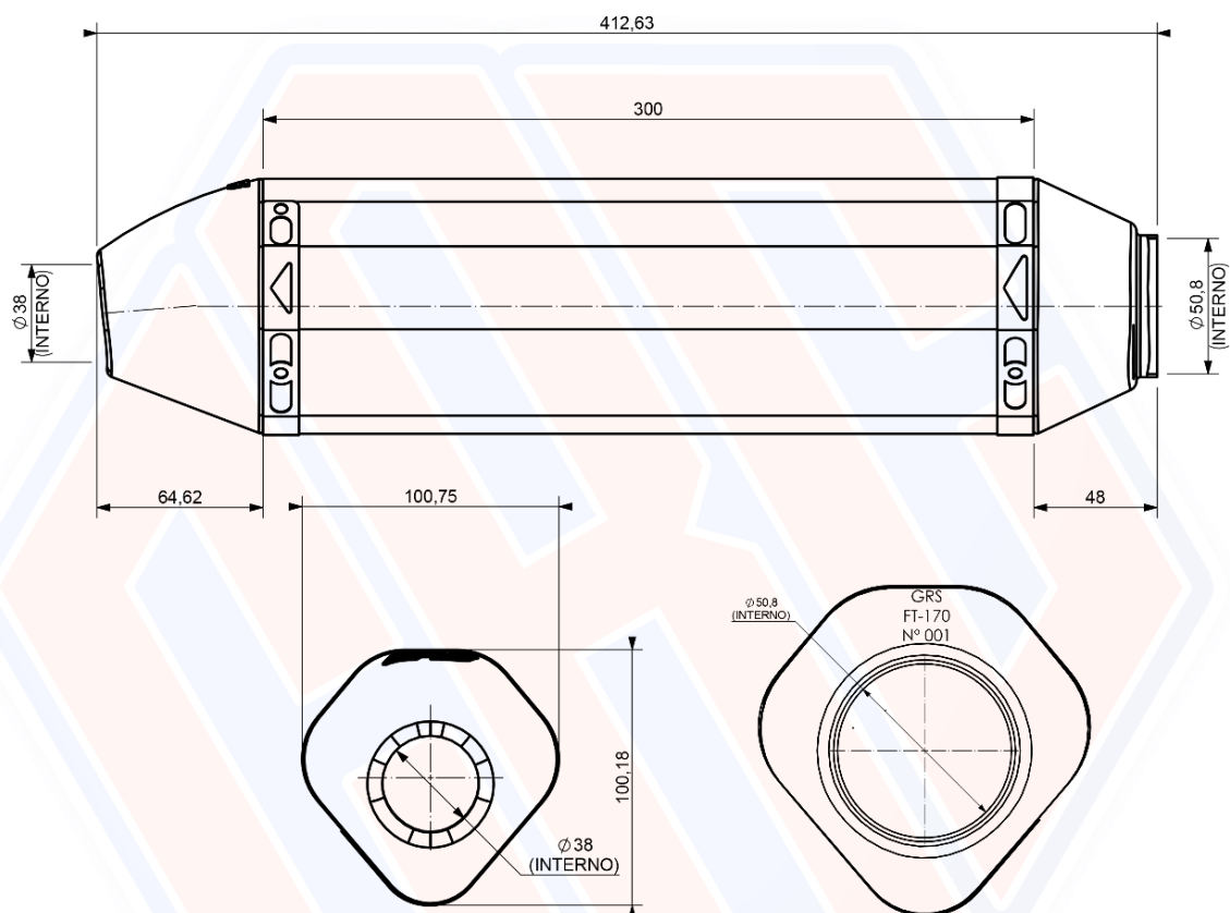
Figura 11 - Desenho Técnico referente ao ARTIGO 37º, PARÁGRAFO 11º
